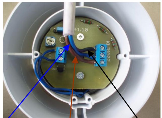
Nulový vodič (N)
